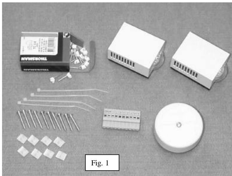
Fig. 1 visar monteringssets innehåll. I satsen finns även 50 meter 4-ledarkabel för givarna.
